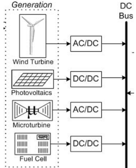
Fig. 6. DER microgrid example.
